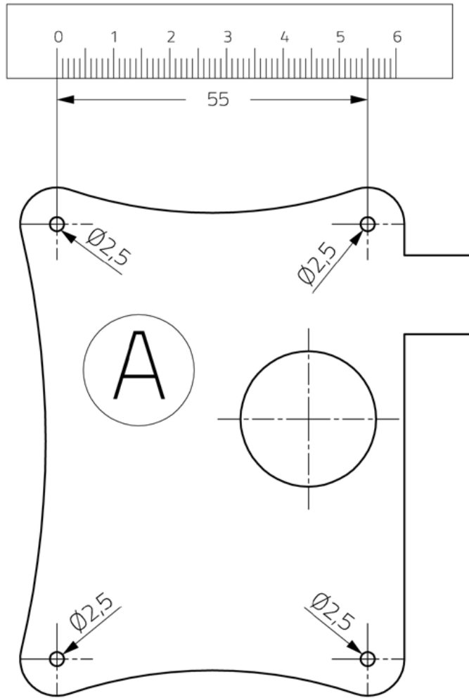
PLANTILLA CERRADURA PUERTA DERECHA TEMPLATE OF RIGHT HAND DOOR
